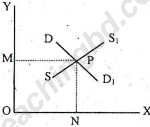
চিত্র: বিনিময় হার নির্ধারণ পদ্ধতি
